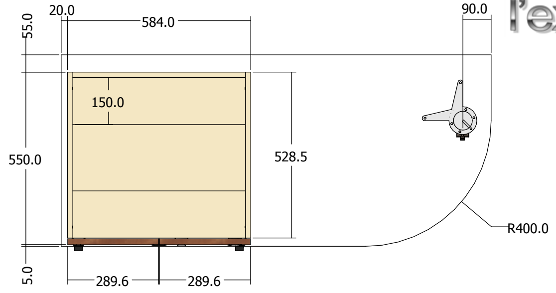
② Plan Caisson 1 : 12
