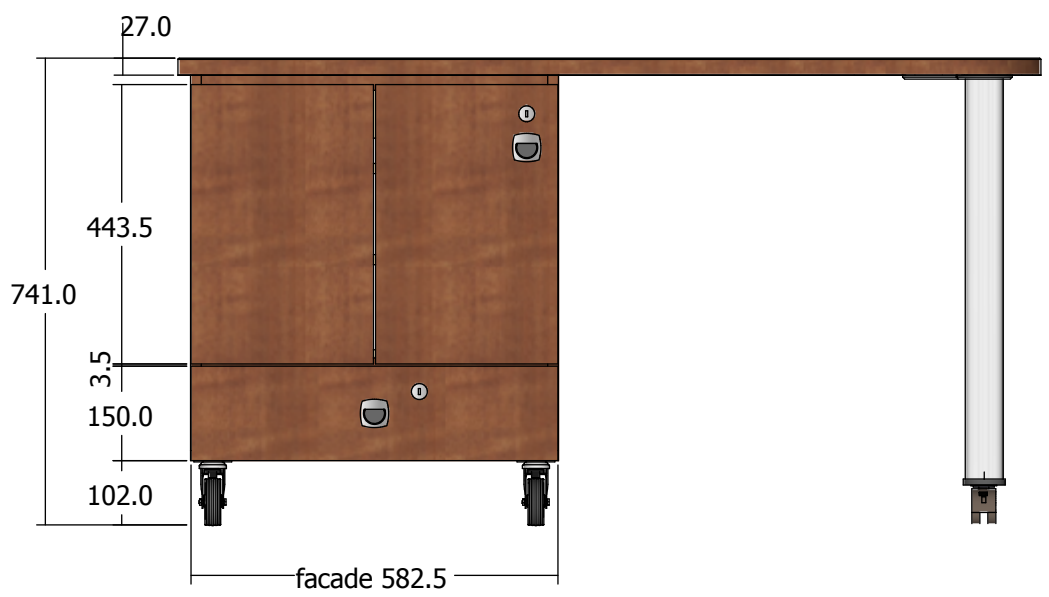
③ Elevation Avant 1 : 12
