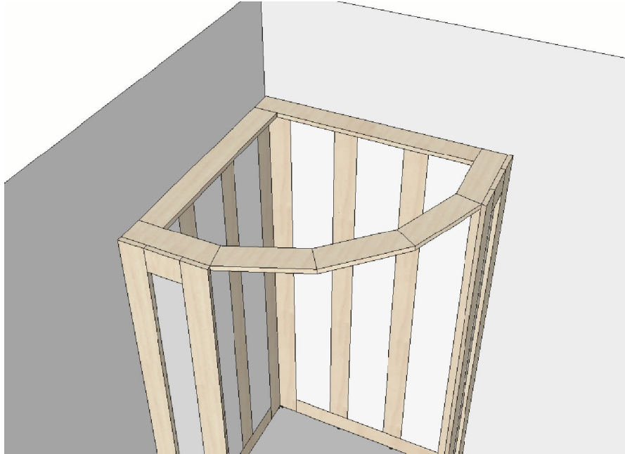
05. Top Frame (7 Pieces)
